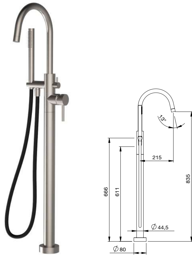
41 512 Grifo exento baño ducha 983 mm redondo con accesorios Floorstanding bath shower mixer 983 mm round with accessories Mitigeur colonne bain douche 983 mm rond avec accessoires напольный смеситель для ванны 983 мм круглый с лейкой
