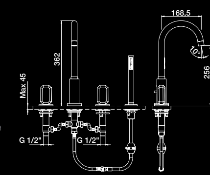
85 714J ● ● ● ● ● ● Grupo baño ducha 4 agujeros de repisa con ducha Bath shower 4 holes mixer with handshower Ensemble bain-douche 4 trous sur gorge avec ensemble de douche Wannenrand bad und duschmischer Смеситель на борт ванны для 4 отверстий с ручным душем
