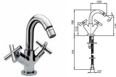
40 009 ● ● Monobloc bidé Single-hole bidet Mélangeur bidet Bidetbatterie Смеситель для Биде
