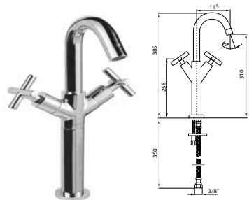
40 102 ● ● Monobloc lavabo alto Single-hole high wash-basin Mélangeur lavabo haut monotrou 1-loch-zweigriff-waschtischbatterie hoher Высокий смеситель для раковины
