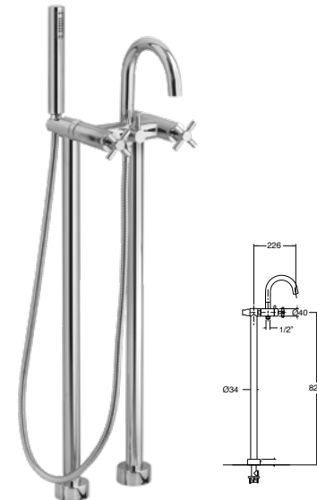
40 512 ● ● Grupo baño ducha con columnas suelo de 800 mm Bath shower group with floor-standing columns of 800 mm Mélangeur bain-douche sur colonnes de 800 mm Wannen batterie mit 800 mm hohen boden anschluss, handbrause und flexiblen schlauch Смеситель ванна / душ с напольными колоннами 800 mm
