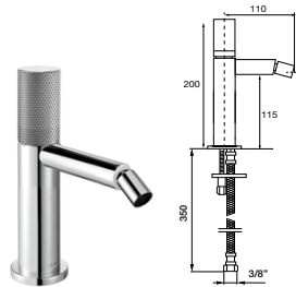
42 009 G1 / G2 ● ● Monomando bidé Bidet mixer Mitigeur bidet Einhebel bidetmischer Однорычажный Смеситель для Биде
