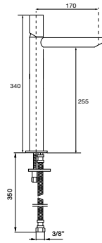
42 102 ●●●●●● Monomando lavabo alto High wash-basin mixer Mitigeur lavabo haut Einhebel waschtischmischer. Hohemn ausführung Однорычажный Смеситель для раковин высокий
