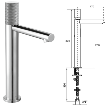
42 102 G1 / G2 ● ● Monomando lavabo alto High wash-basin mixer Mitigeur lavabo haut Einhebel waschtischmischer. Hohemn ausführung Однорычажный Смеситель для раковин высокий
