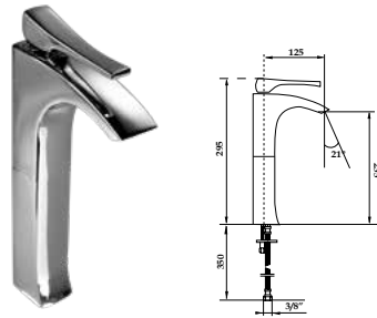
58 102 ● ● ● ● Monomando lavabo alto High wash-basin mixer Mitigeur lavabo haut Einhebel waschtischmischer. Hohemrn ausführung Однорычажный Смеситель для раковин высокий
